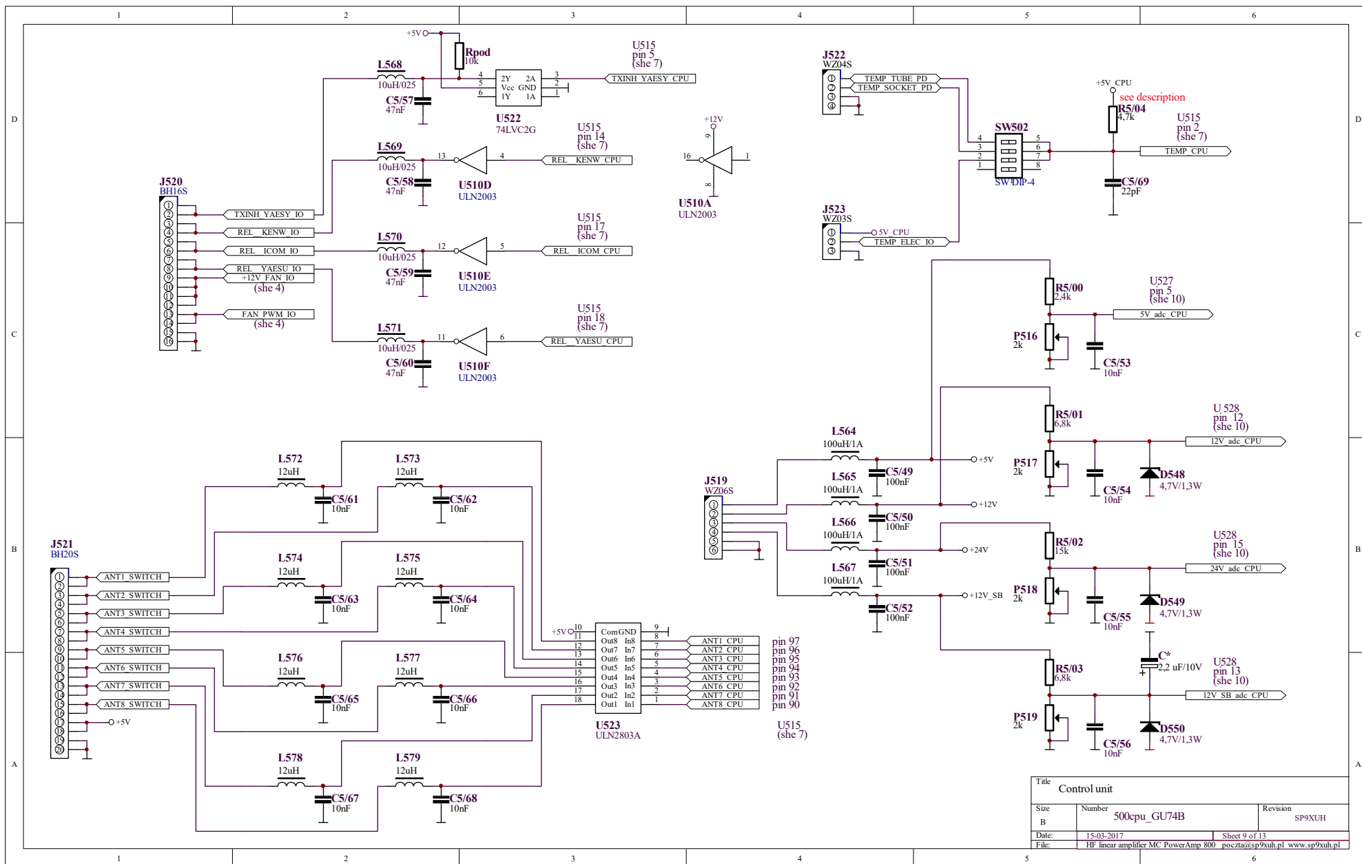
Schemat 7-9 500cpu_she9 - jednostka centralna – pomiary, sterowanie przełącznika antenowego
