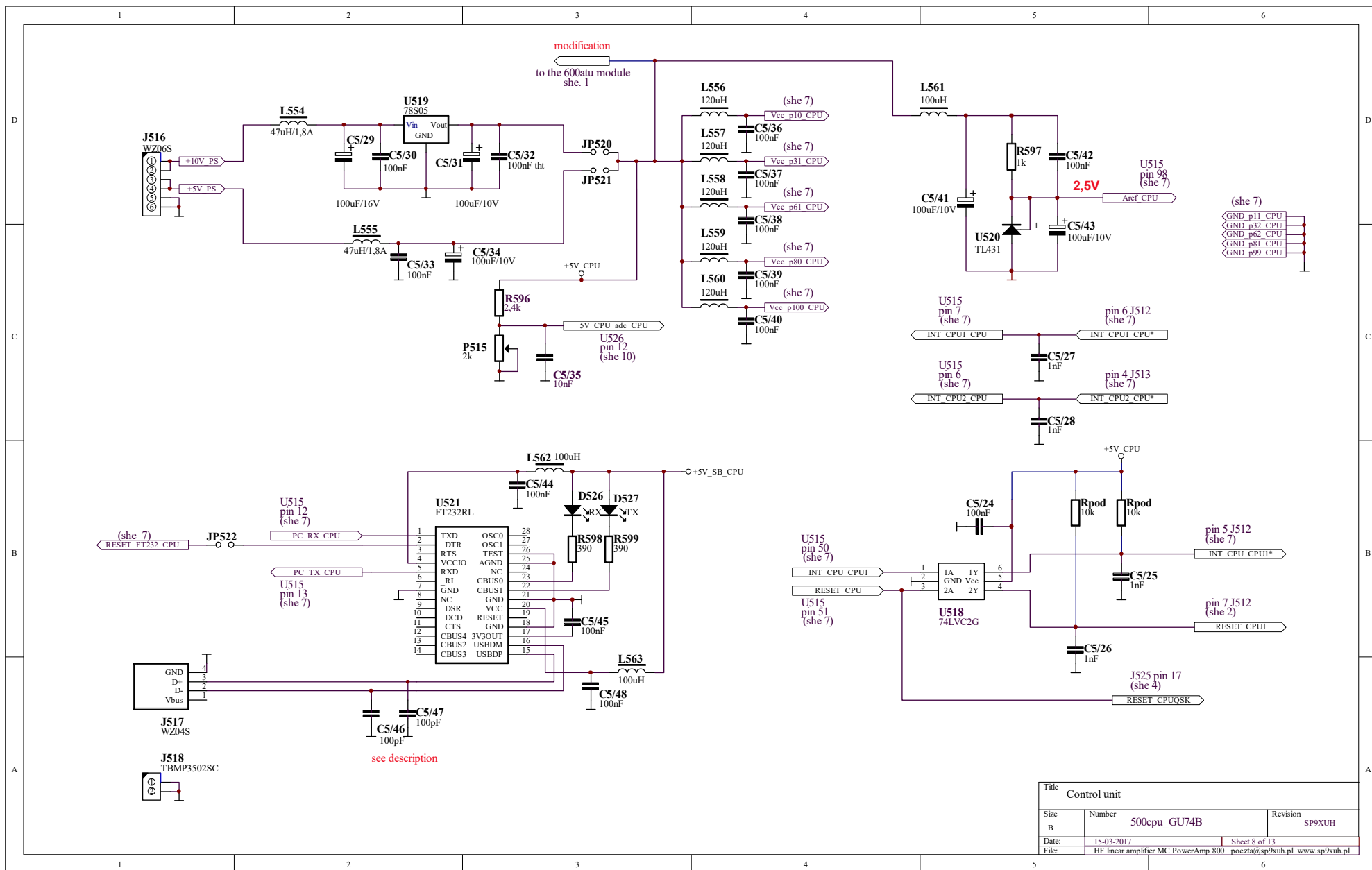
Schemat 7-8 500cpu_she8 - jednostka centralna – zasilanie, konwerter USB/RS232.
