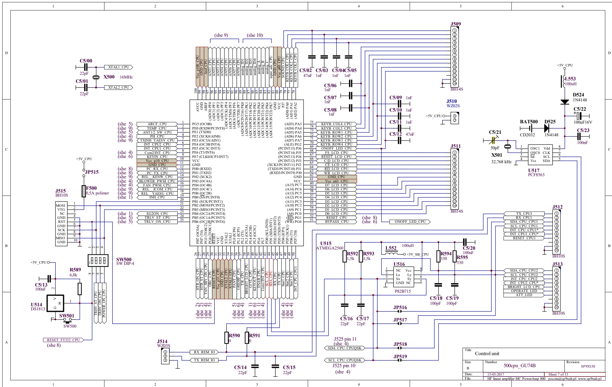
Schemat 7-7 500cpu_she7 - jednostka centralna – procesor.
