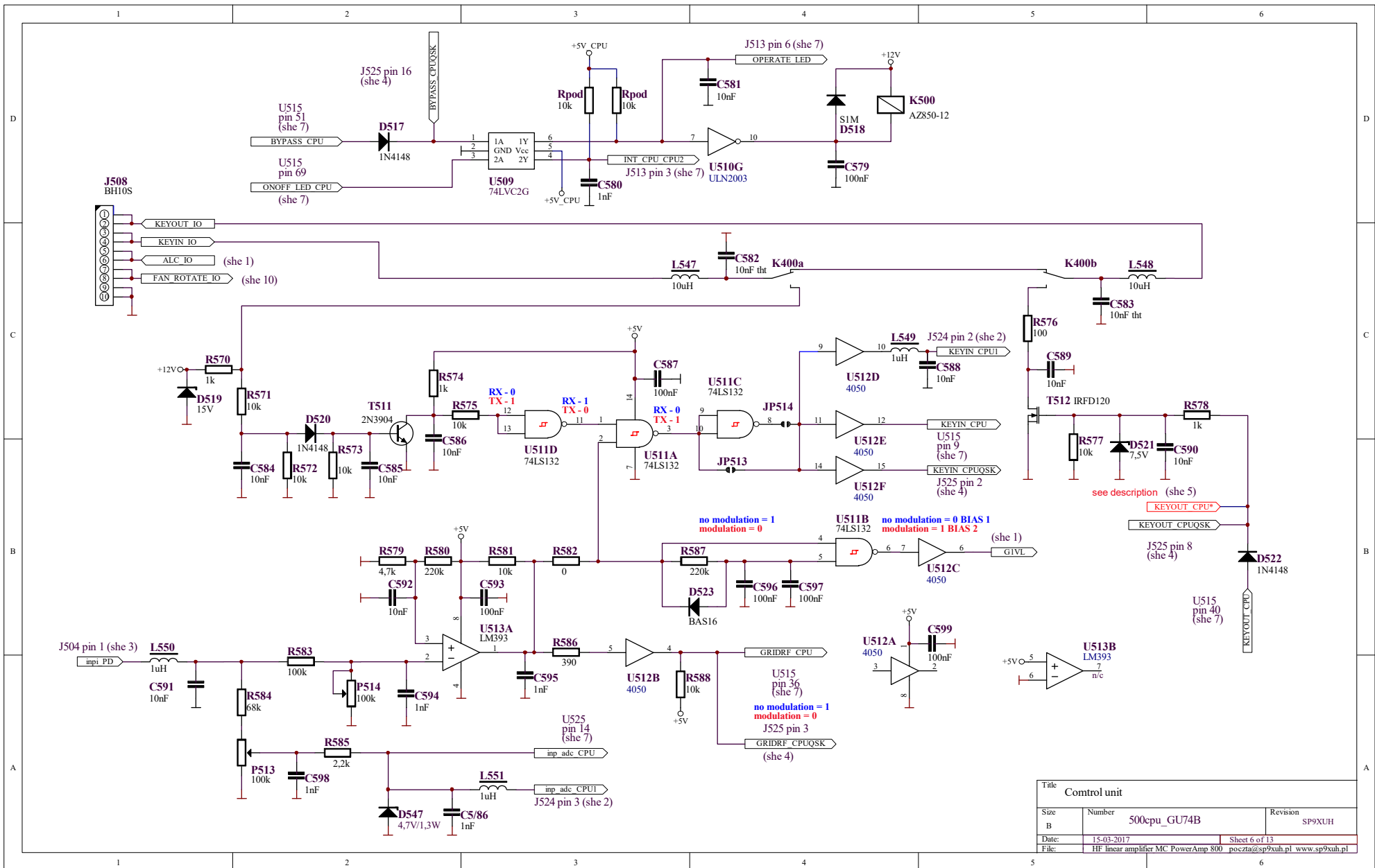
Schemat 7-6 500cpu_she6 - jednostka centralna – przełączanie NAD/ODB.
