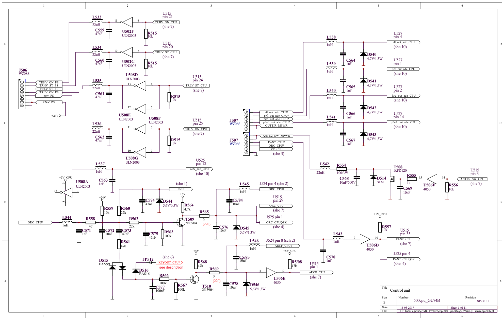
Schemat 7-5 500cpu_she5 - jednostka centralna – ORC, ARCF, pomiary, sterowanie.
