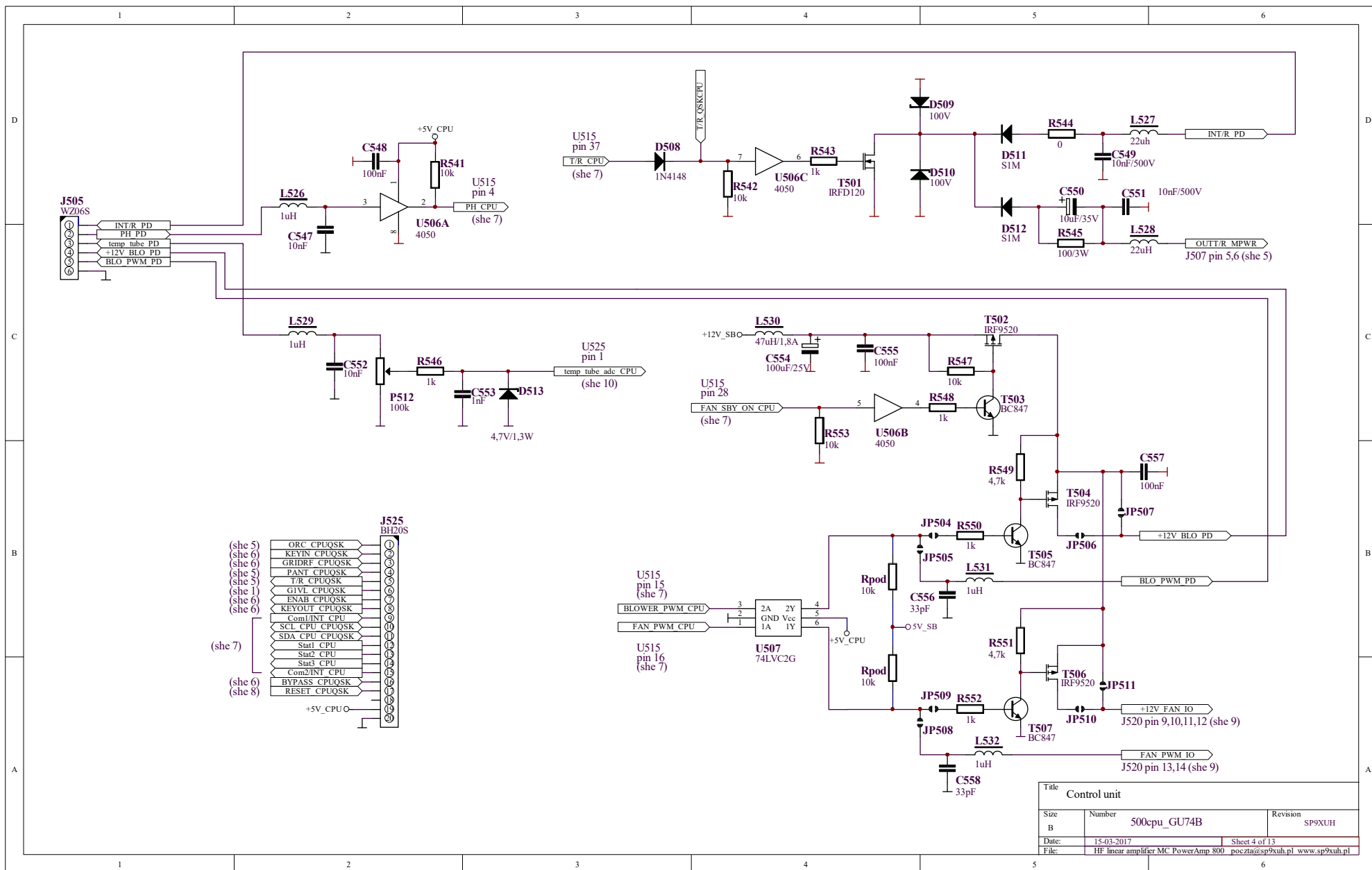
Schemat 7-4 500cpu_she4 - jednostka centralna – przełączenie NAD/ODB, układ chłodzenia.
