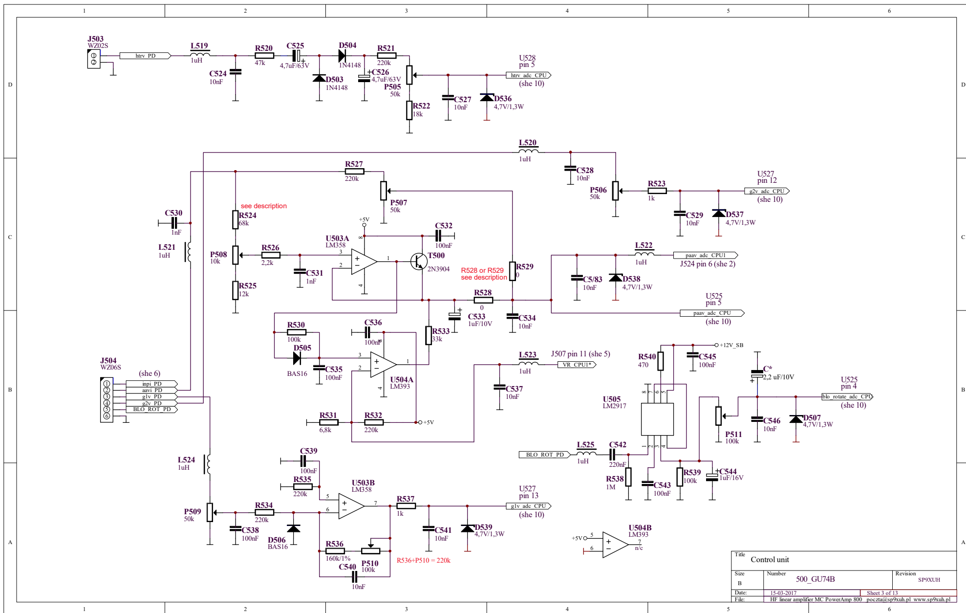
Schemat 7-3 500cpu_she3 - jednostka centralna – pomiary.
