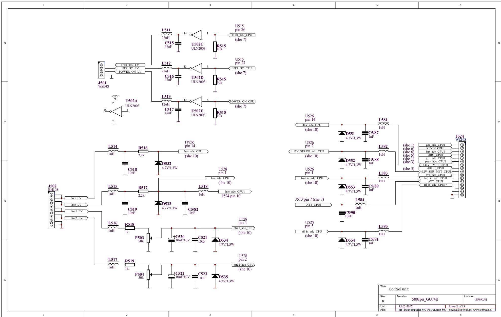
Schemat 7-2 500cpu_she2 - jednostka centralna - pomiary, sterowanie.
