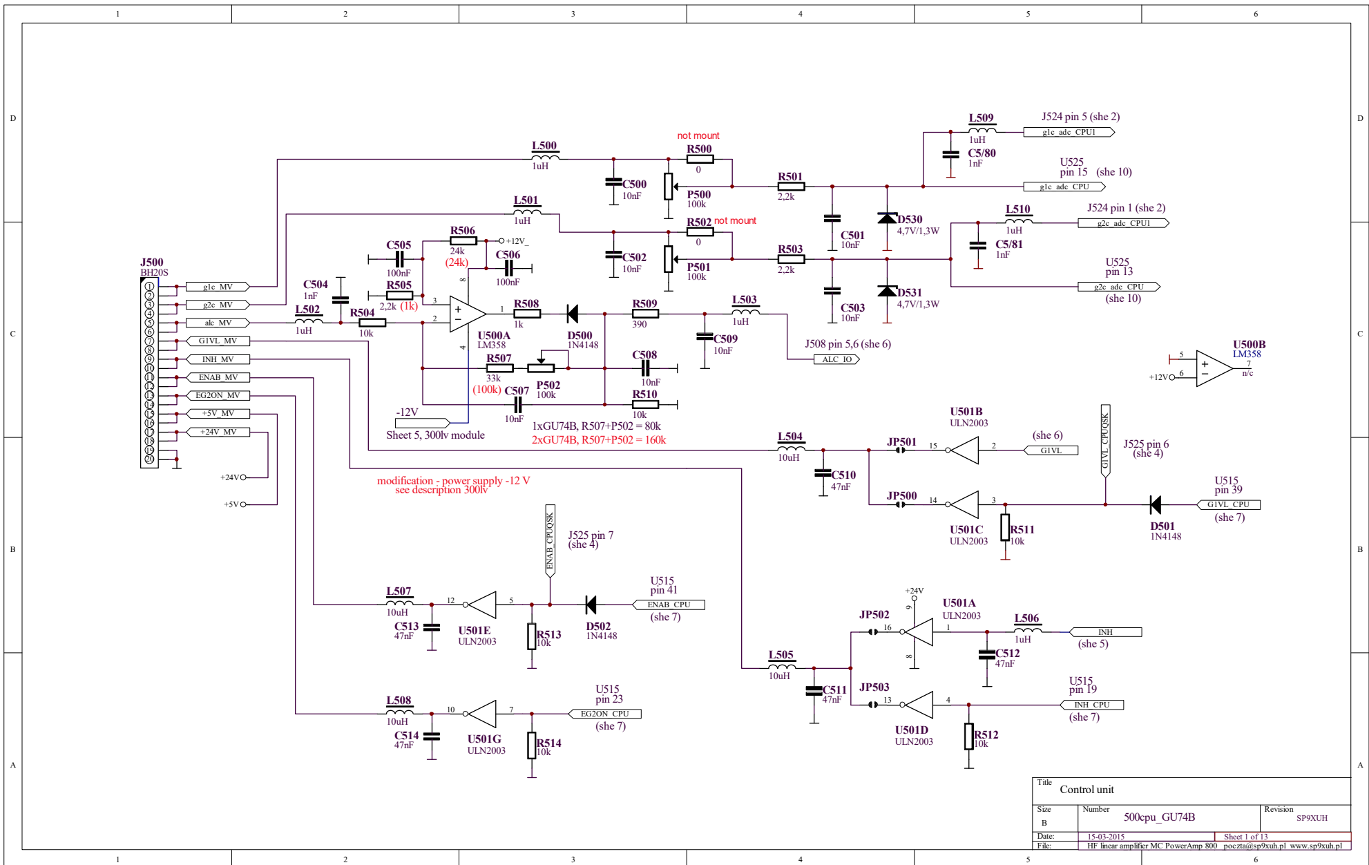
Schemat 7-1 500cpu_she1 - jednostka centralna - ALC, pomiary, sterowanie.
