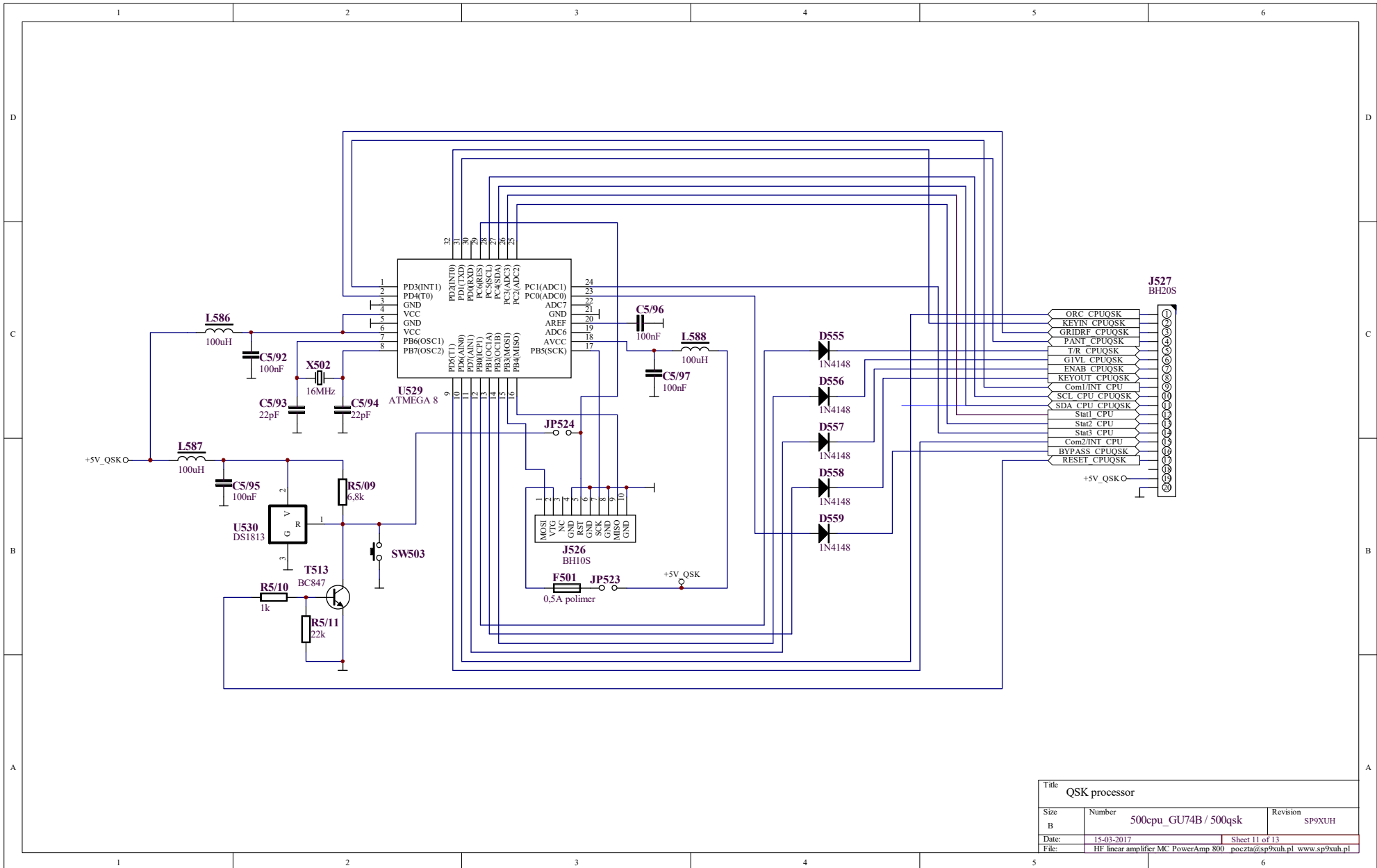
Schemat 7-11 500cpu_she11 - procesor QSK.
