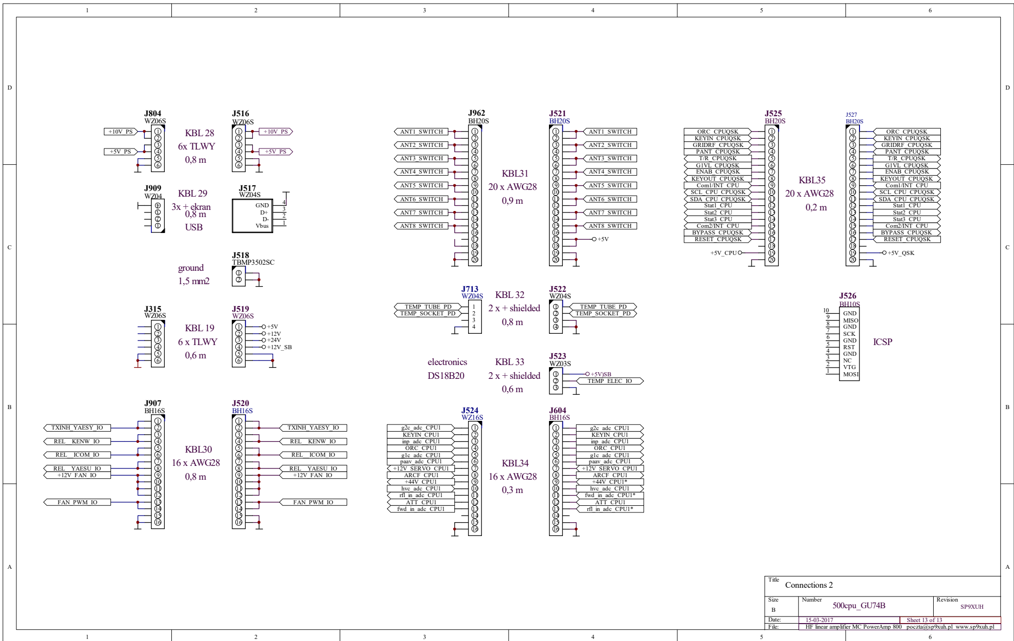
Schemat 7-13 500cpu_con2 - jednostka centralna, część 2.
