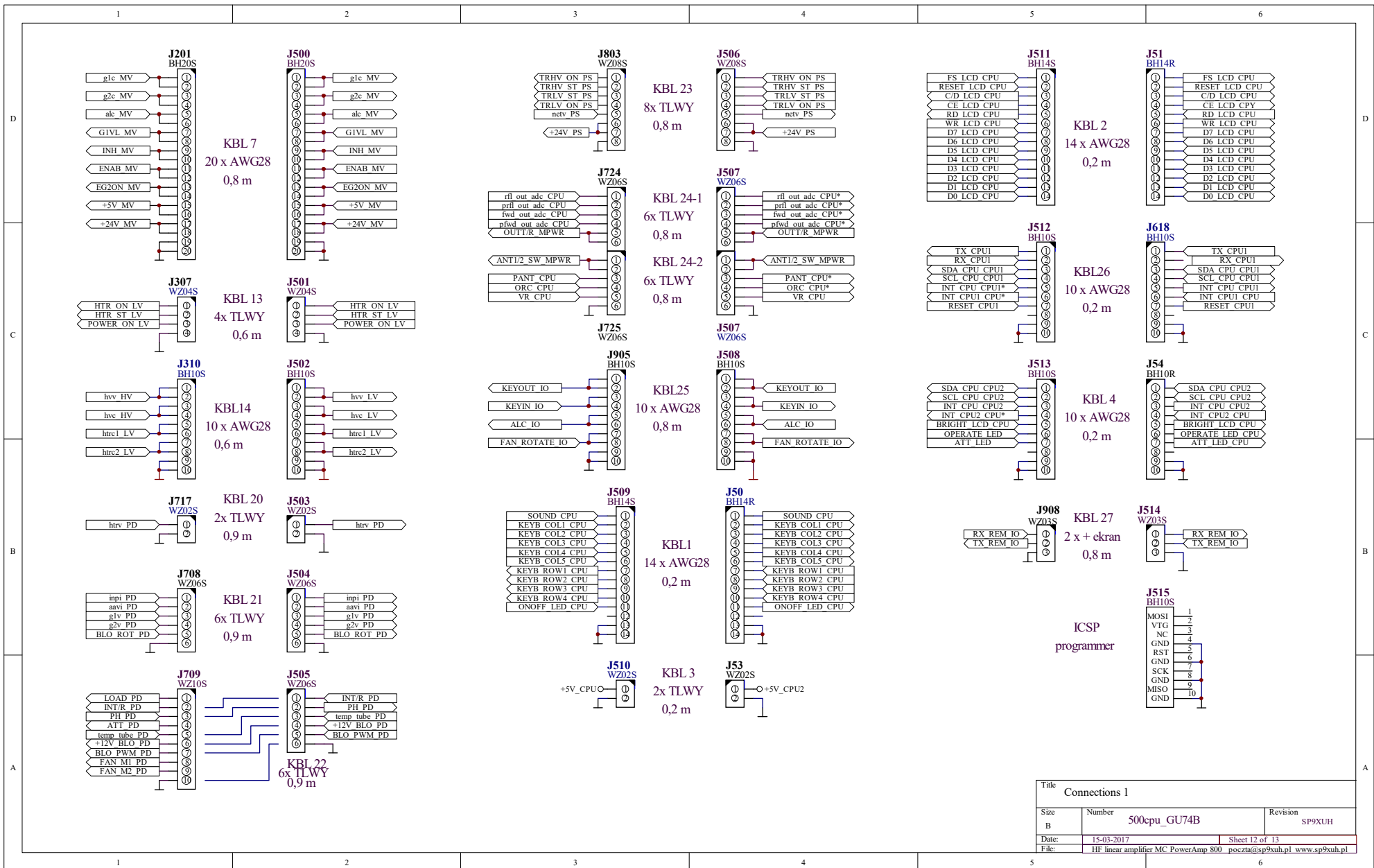
Schemat 7-12 500cpu_con1 - jednostka centralna, część 1.
