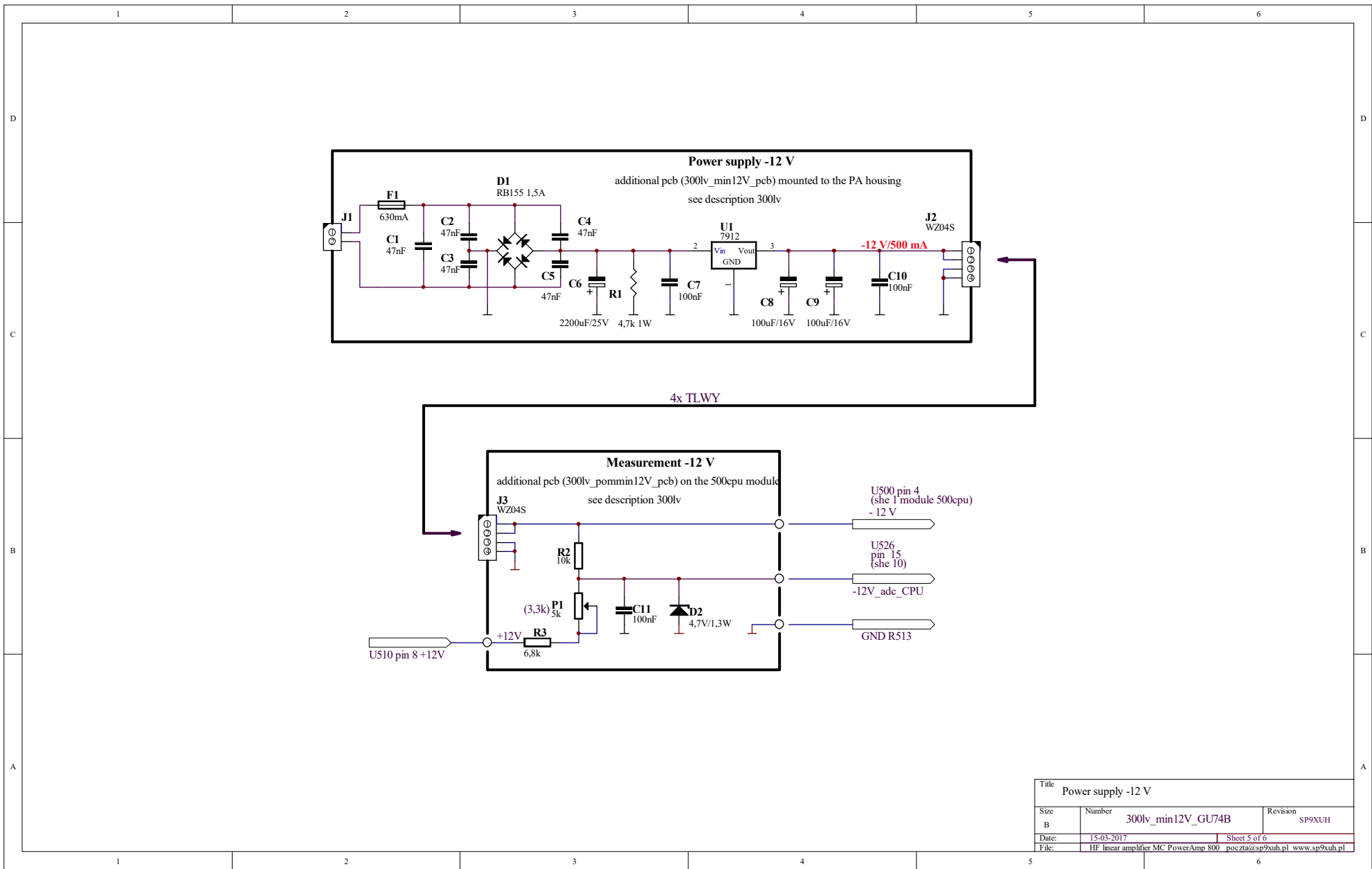
Schemat 6-5 300lv_she5 - zasilacz i pomiar napięcia -12V.
