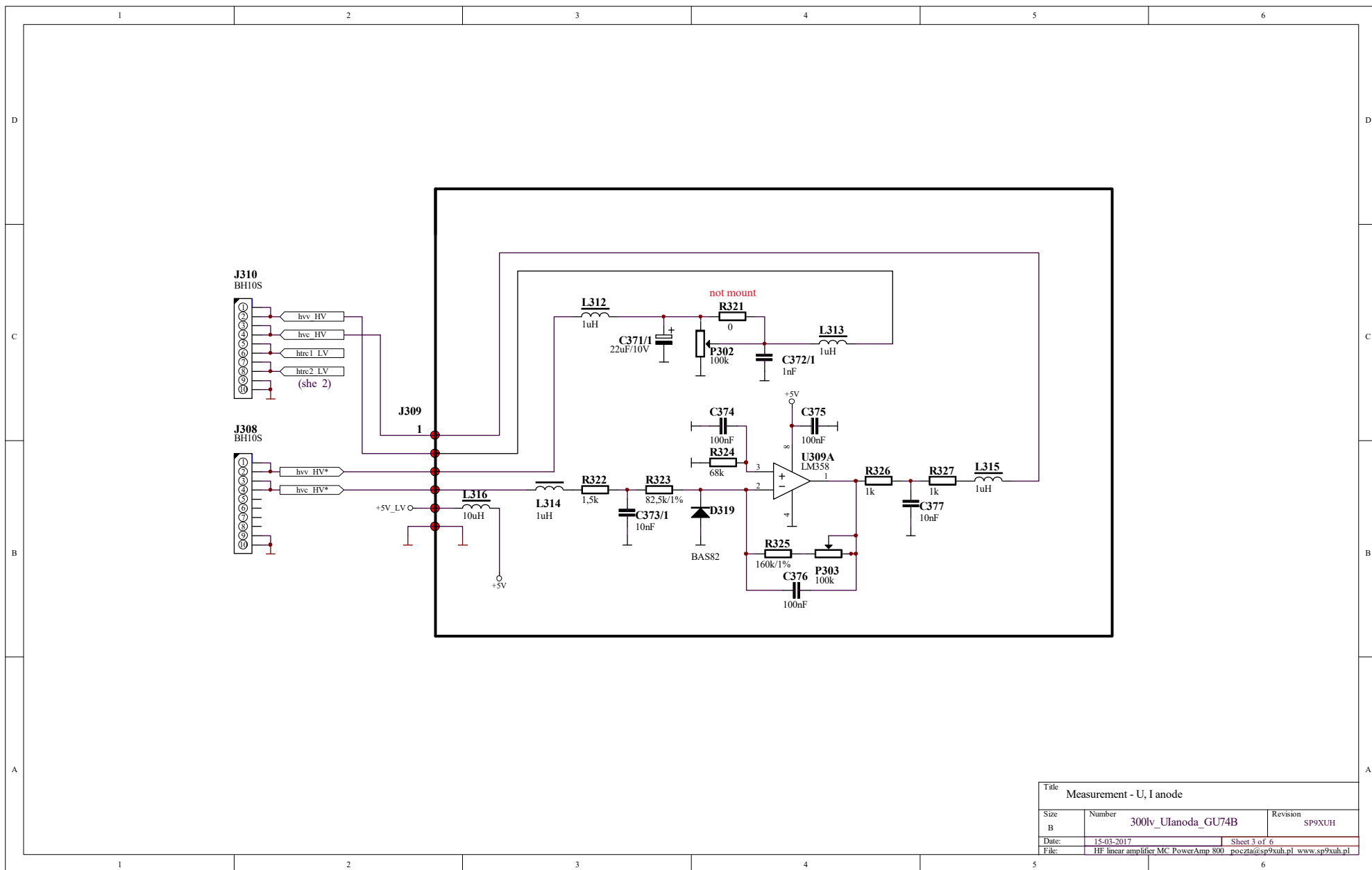
Schemat 6-3 300lv_she3 - pomiar napięcia i prądu anody (sub-moduł).
