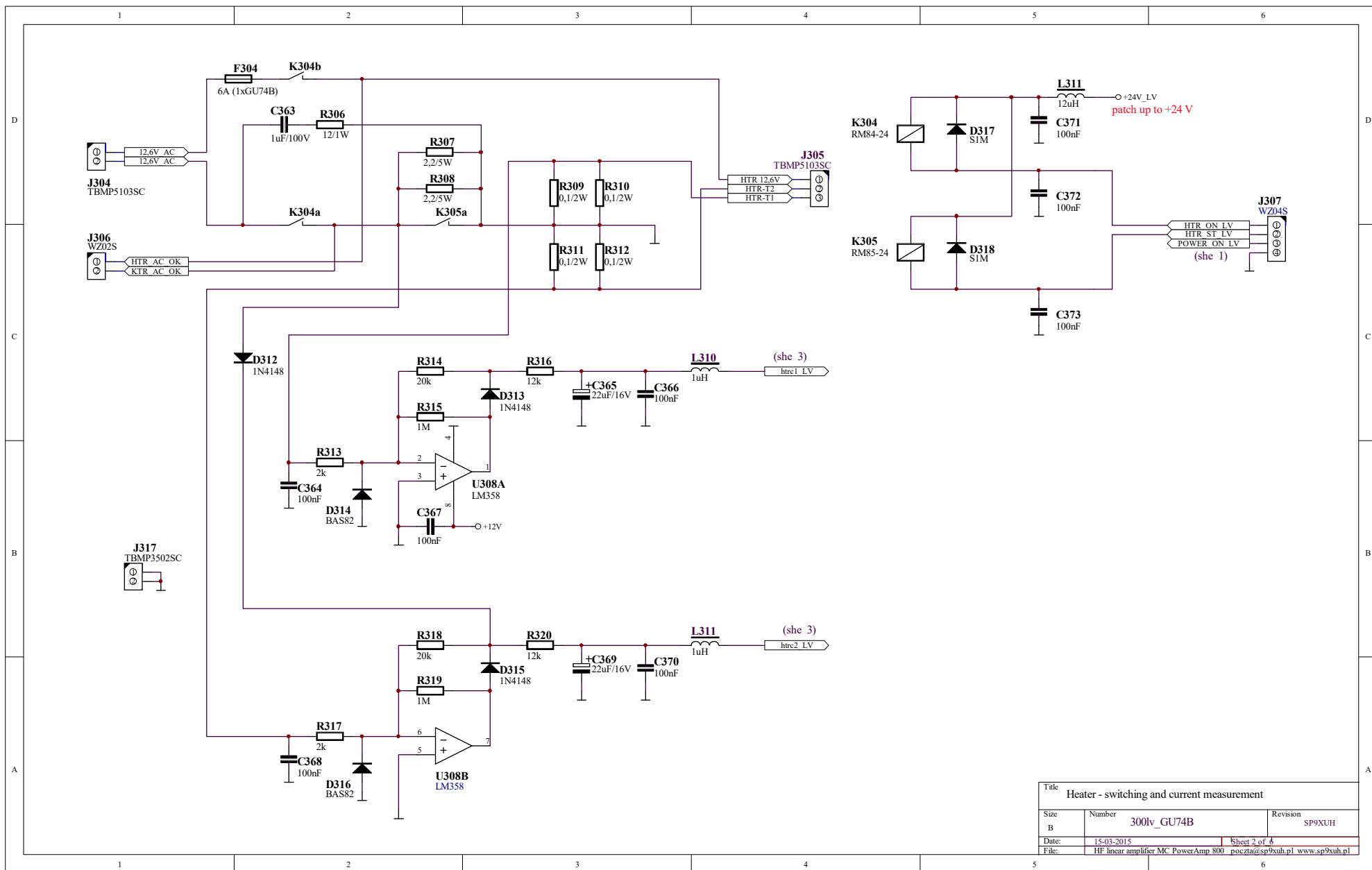
Schemat 6-2 300lv_she2 - załączanie żarzenia i pomiar prądu żarzenia.
