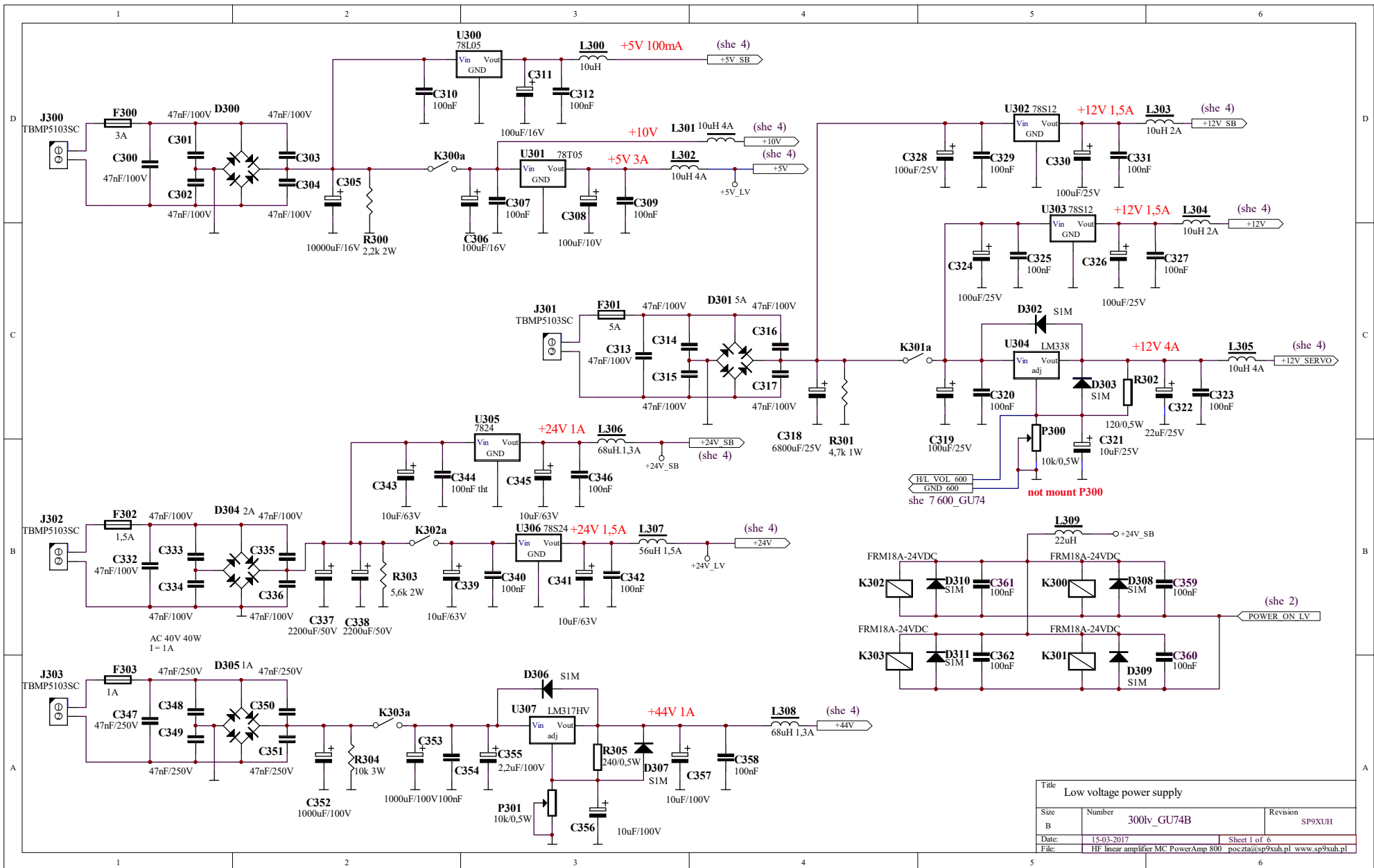
Schemat 6-1 300lv_she1 - zasilacze: +5V, +12V, +24V, +44V.
