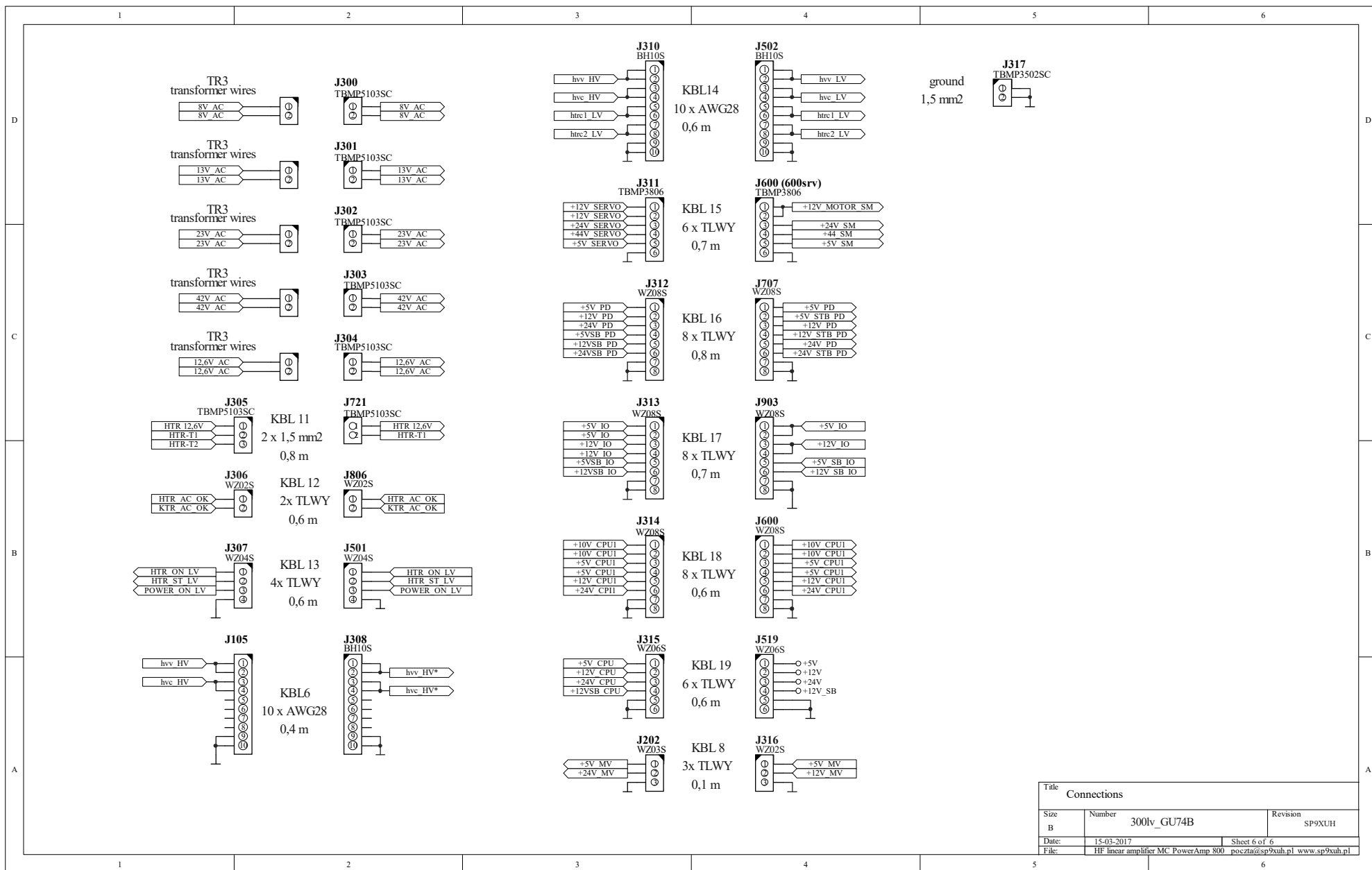
Schemat 6-6 300lv_con - połączenia, zasilacze niskich napięć.
