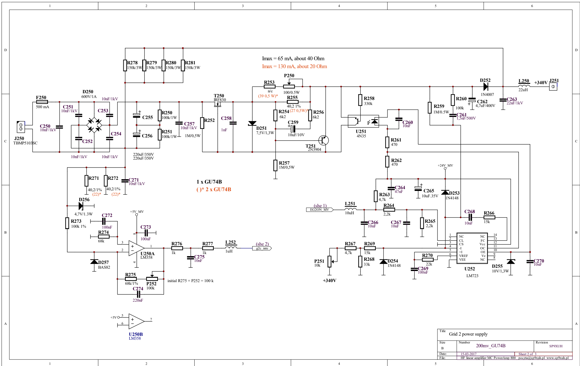
Schemat 5-2 200mv_she2 - zasilacz siatki przyspieszającej +340 V
