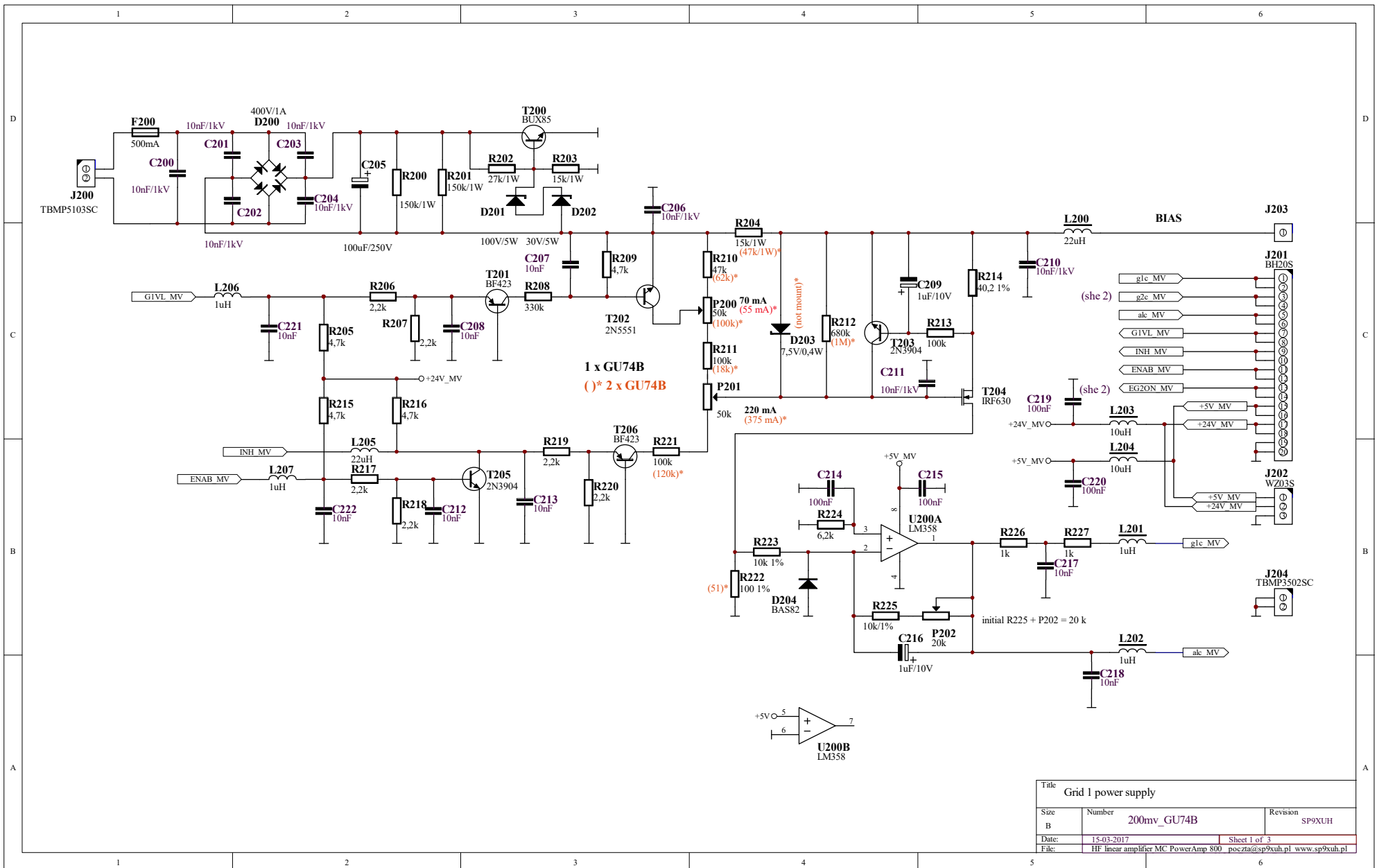
Schemat 5-1 200mv_she1 - zasilacz siatki sterującej –130 V.
