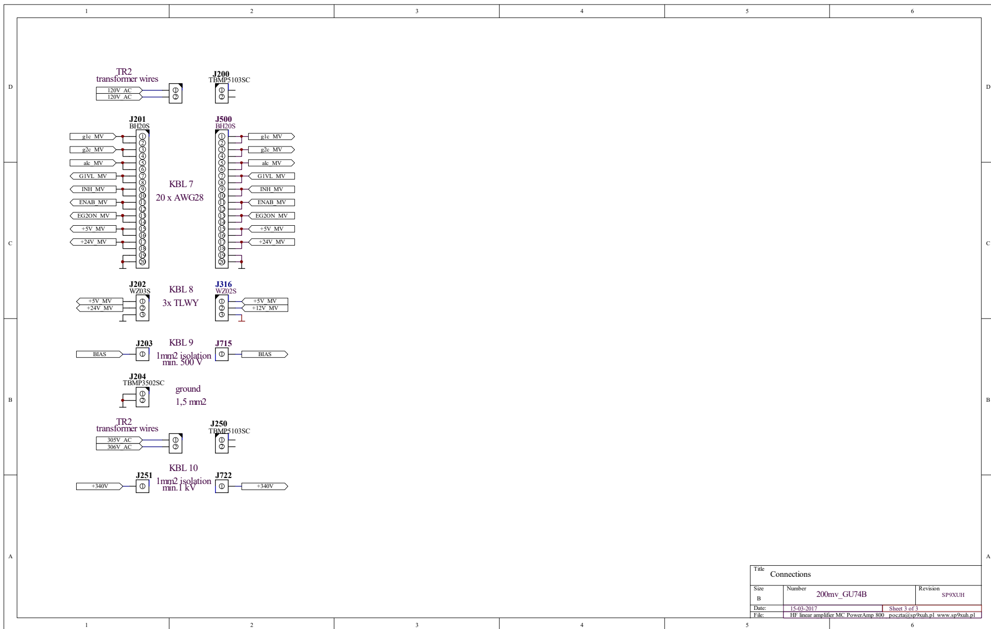
Schemat 5-3 200mv_con, połączenia - zasilacz średnich napięć.
