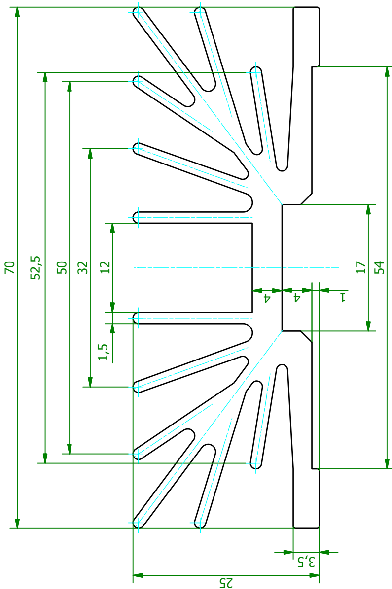
Rysunek G-5-2 Radiator 70x25 mm.
