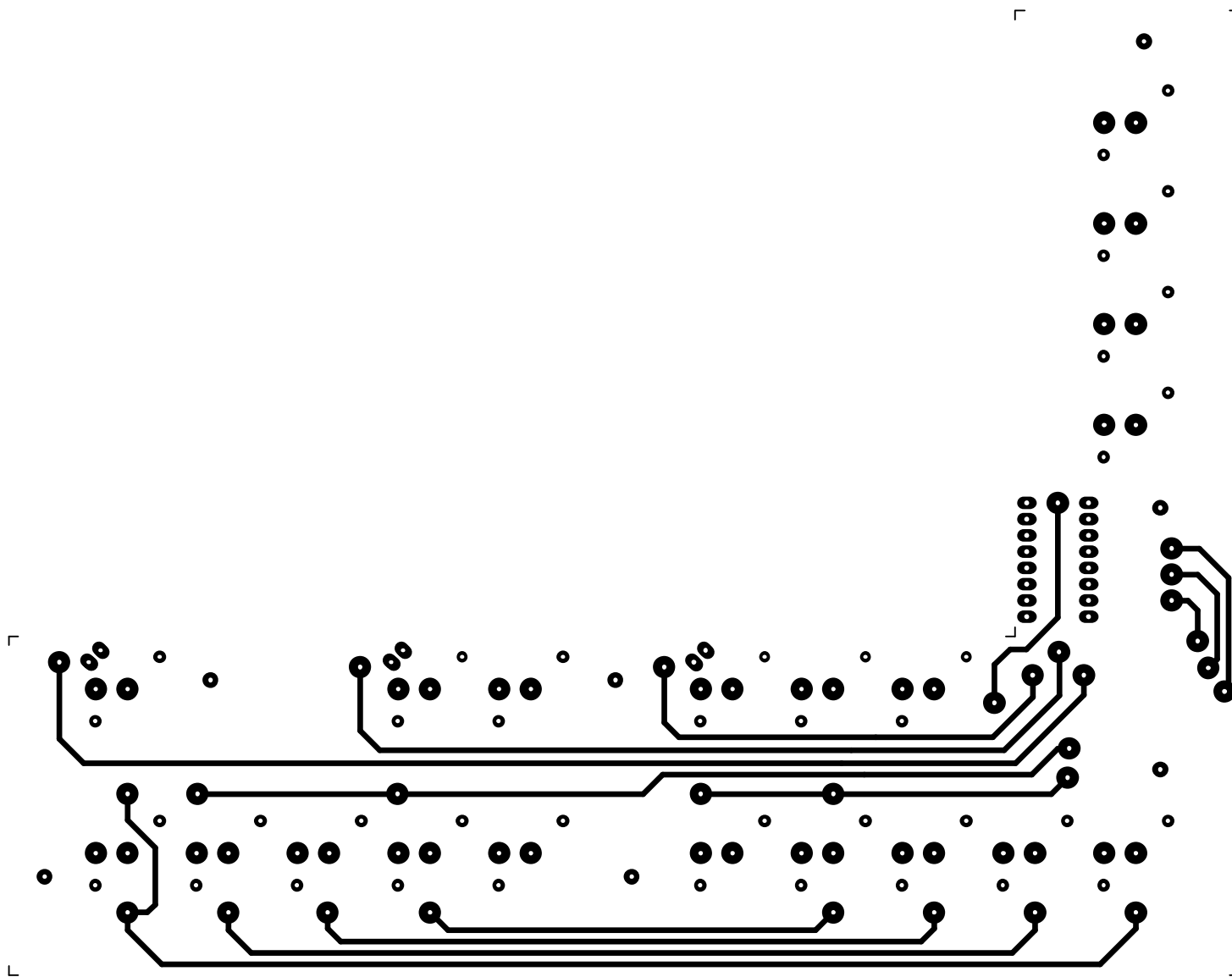
Płytko 3-5 50disp, klawiatura, odbicie lustrzane – góra płytki
