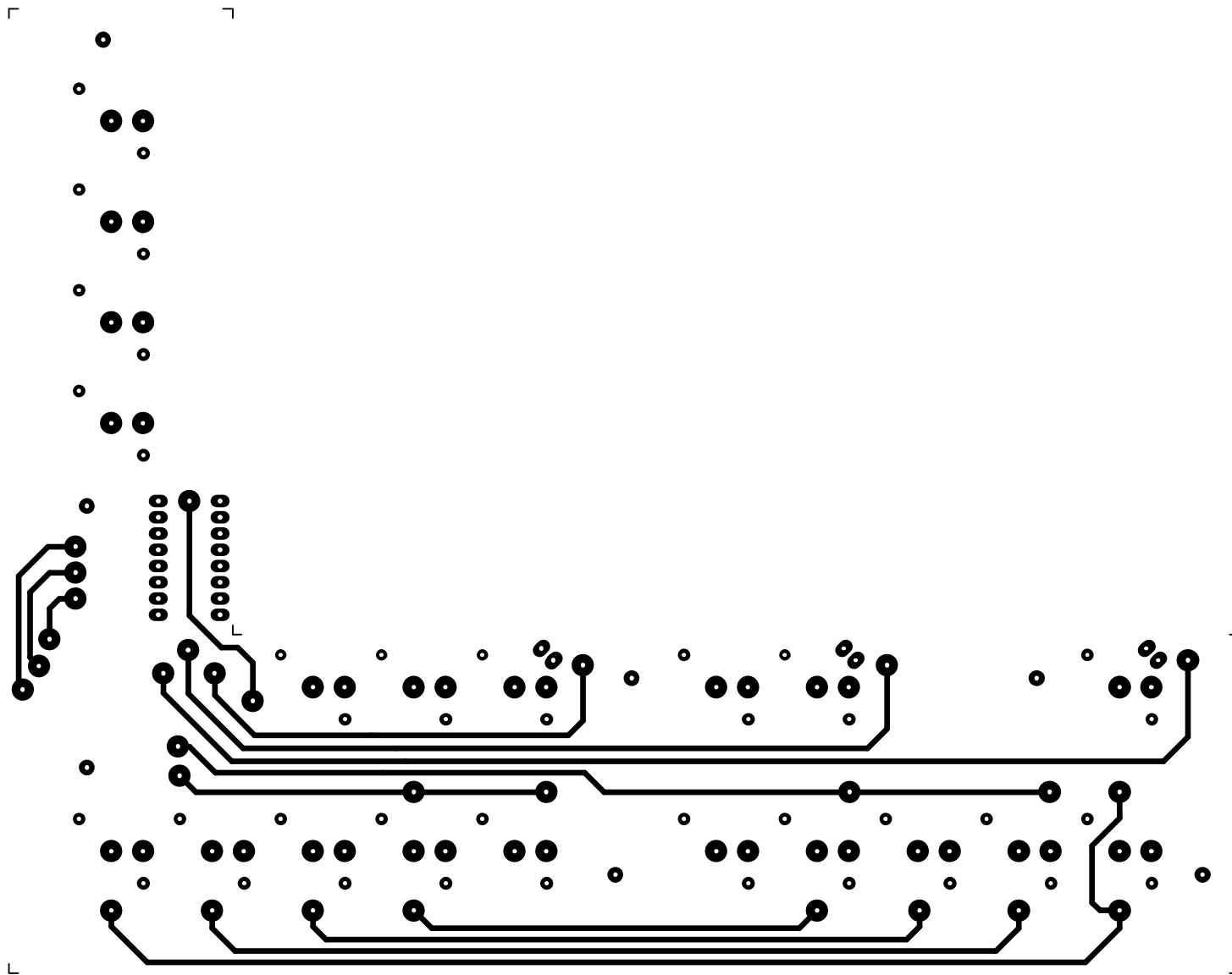
Płytki 3-1 50disp, klawiatura – góra płytki
