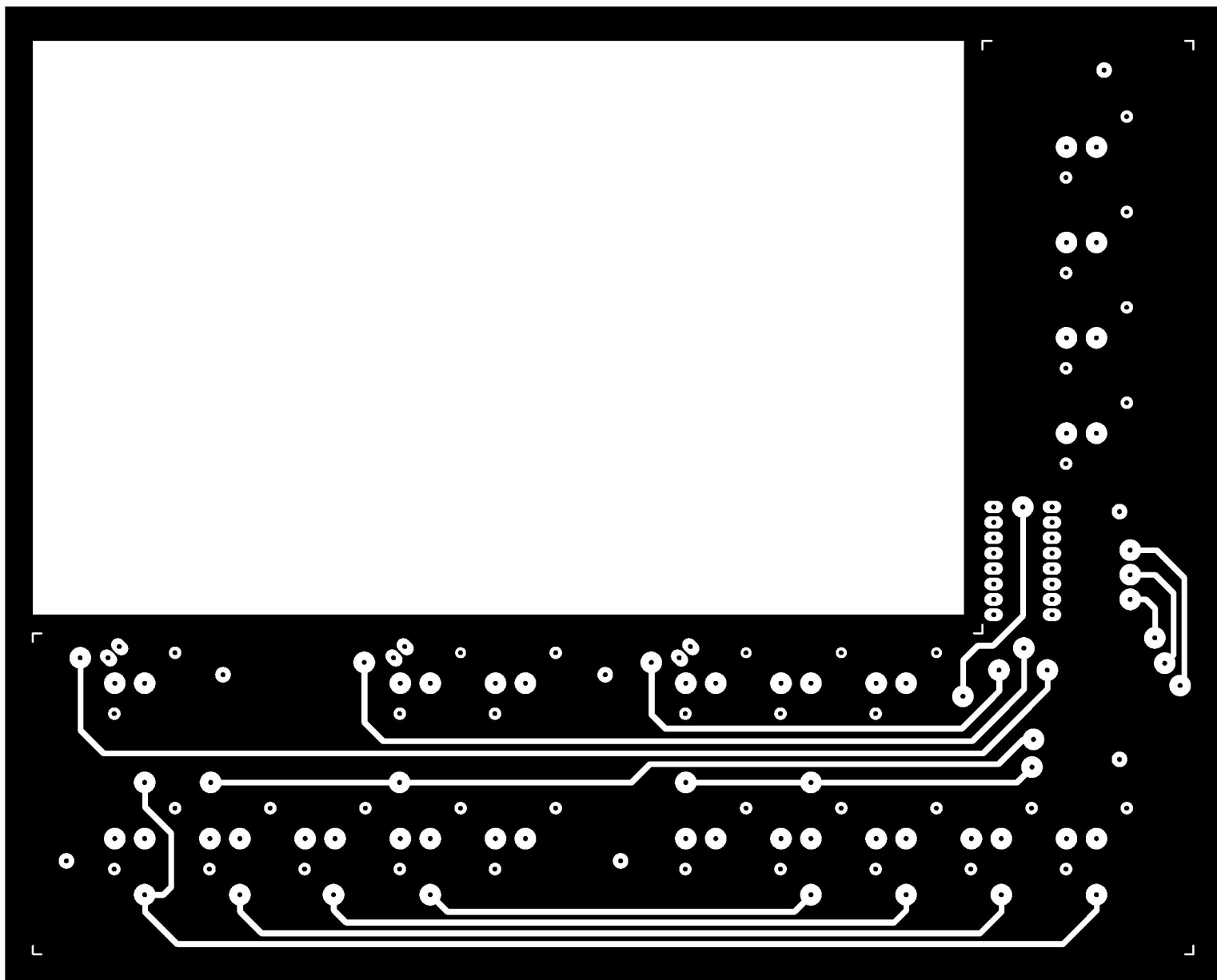
Płytką 3-3 50disp, klawiatura, negatyw, odbicie lustrzane (MIRROR) – góra płytki
