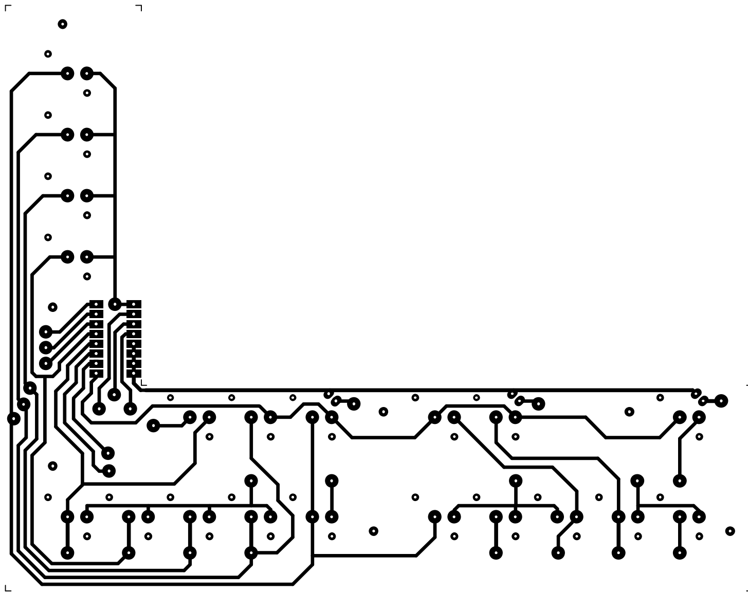
Płytki 3-6 50disp, klawiatura, odbicie lustrzane – spód płytki
