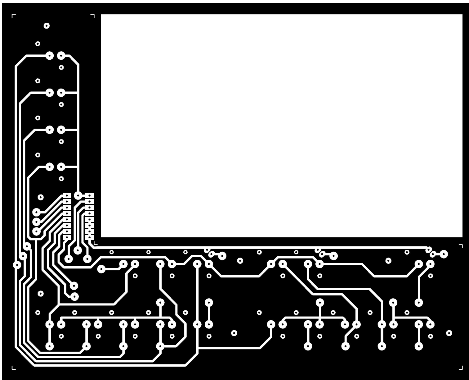
Płytki 3-4 50disp, klawiatura, negatyw, odbicie lustrzane (MIRROR) – spód płytki
