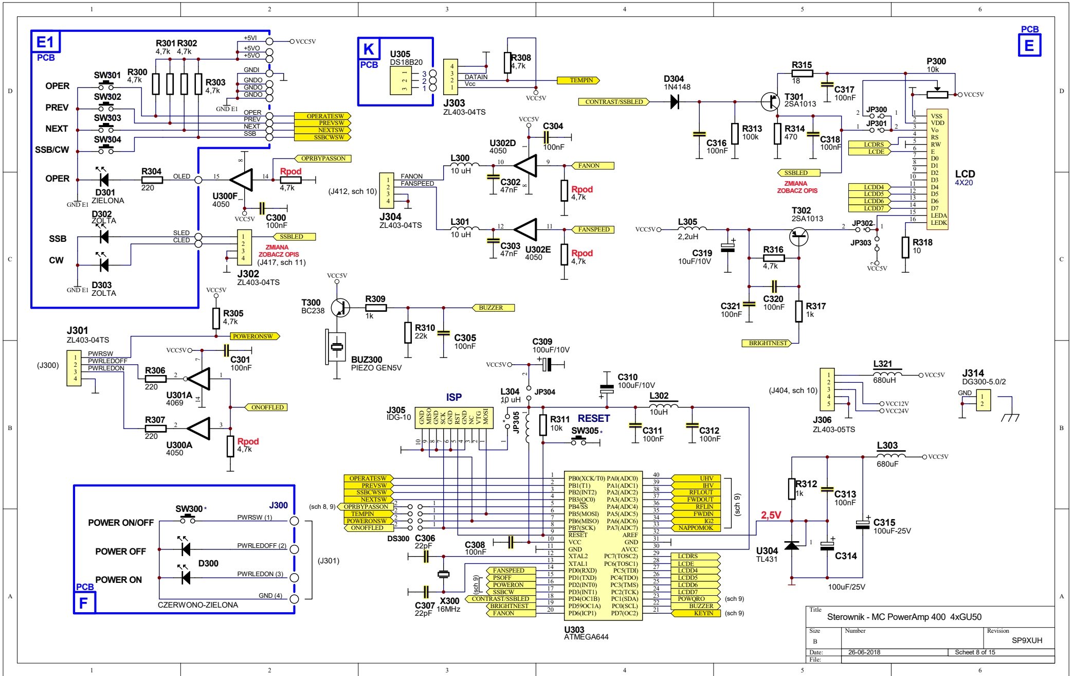
Schemat 8 - Sterownik mikroprocesorowy.
