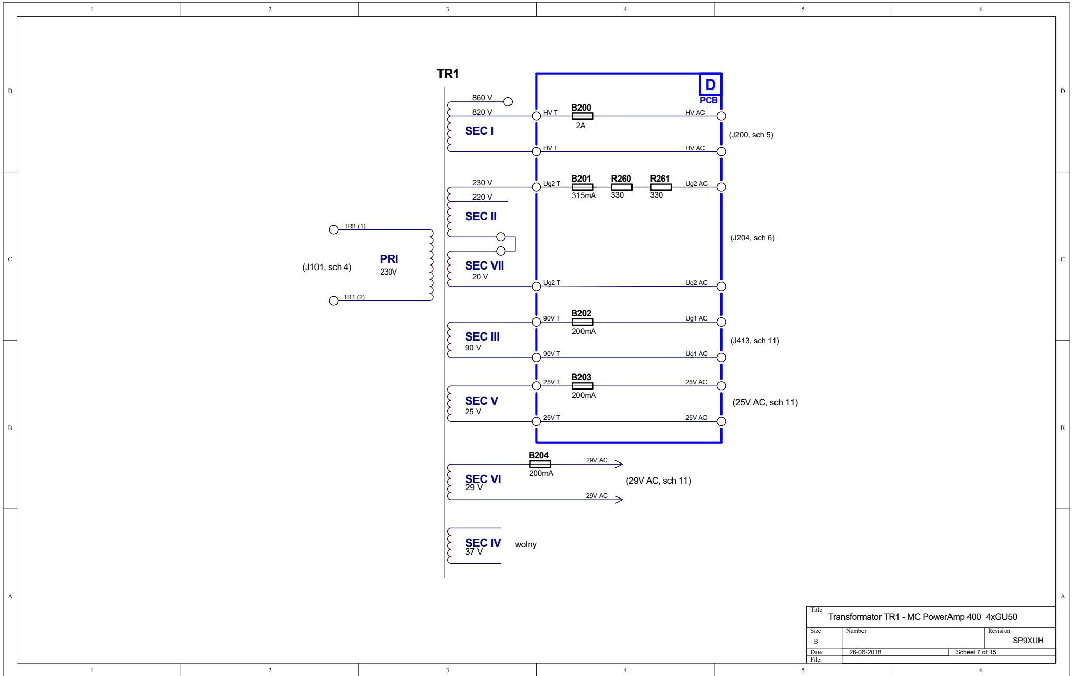
Schemat 7 - Transformator TR1, bezpieczniki.
