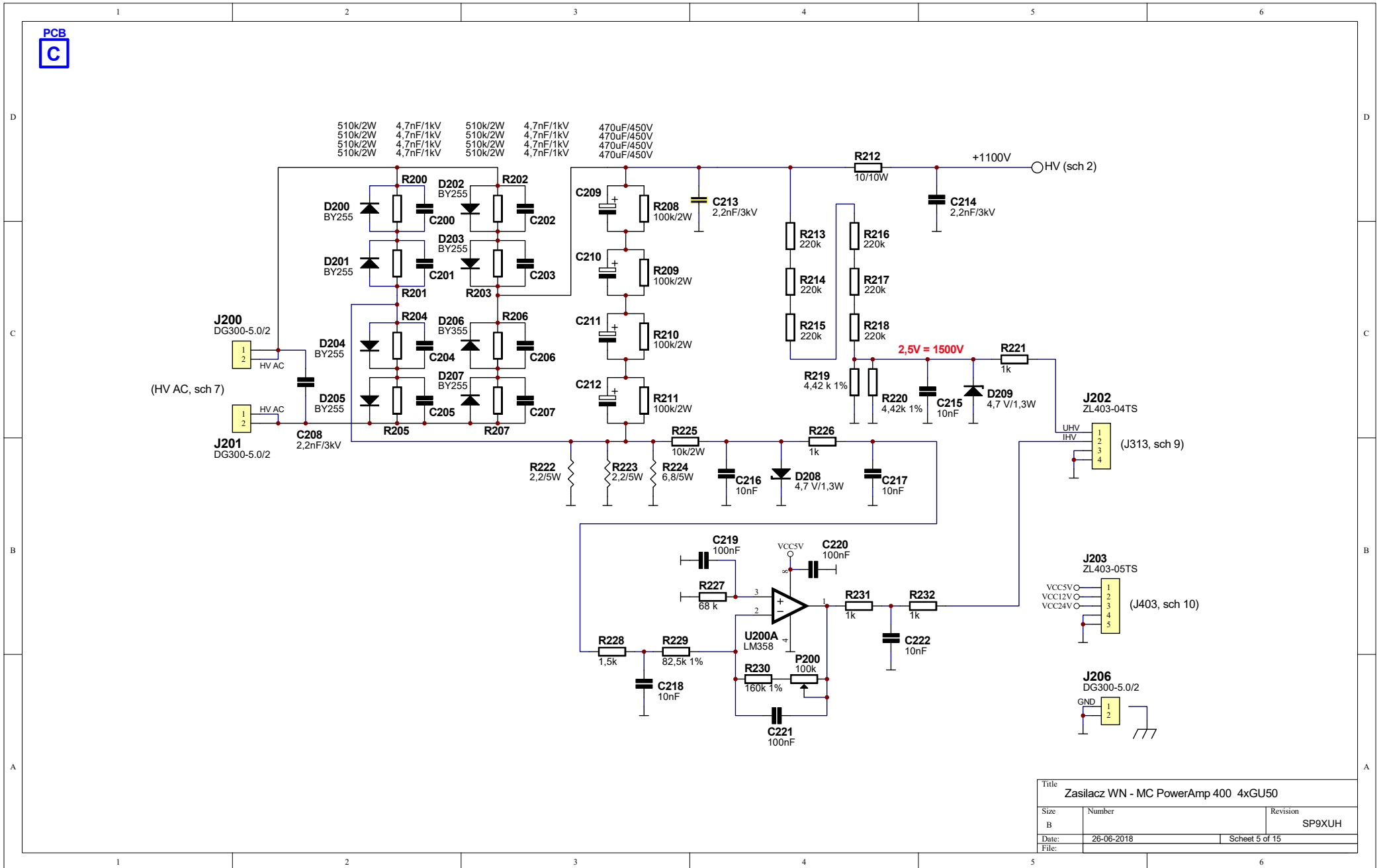
Schemat 5 - Zasilacz napięcia anody.
