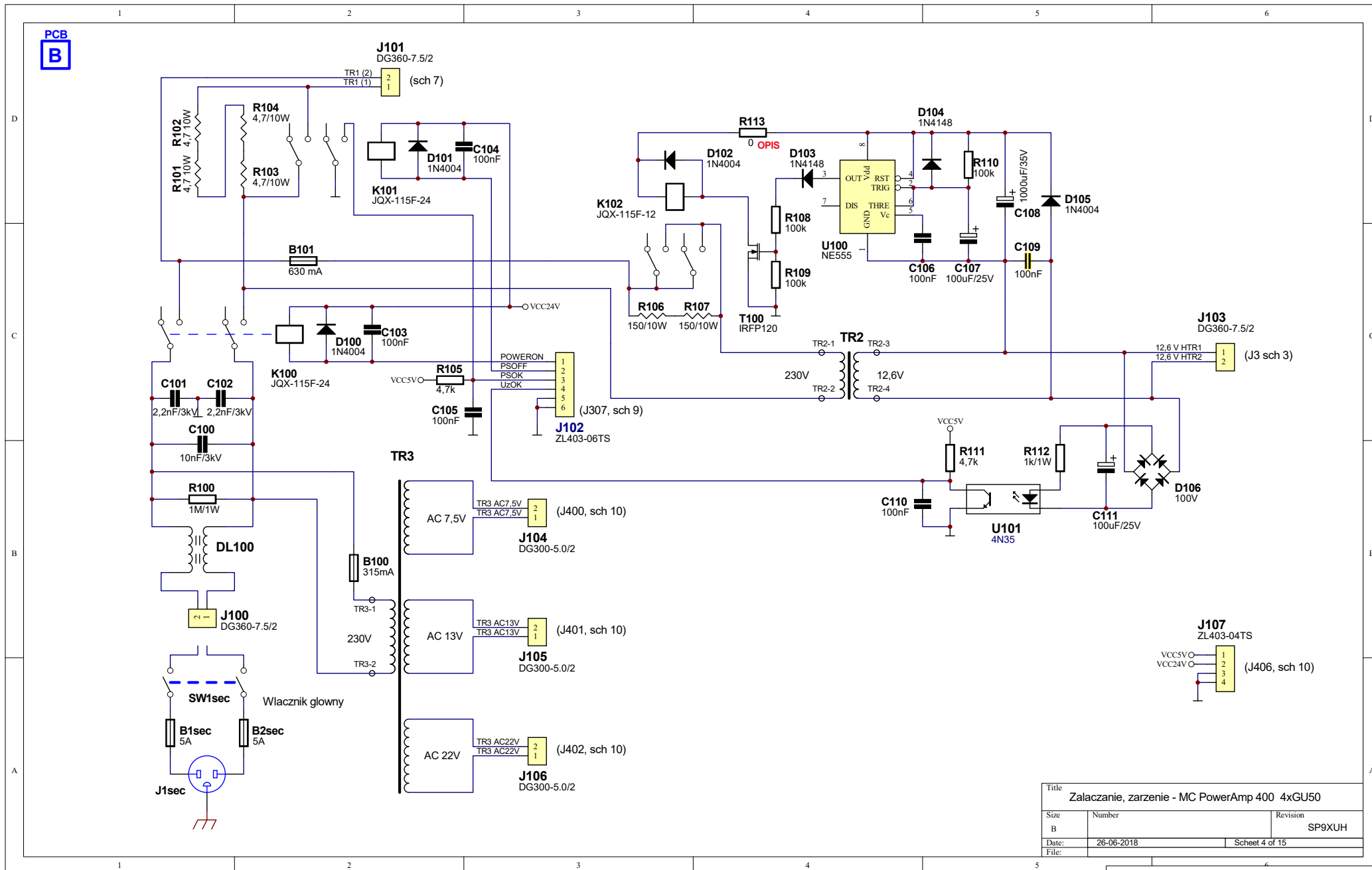
Schemat 4 - Zalaczenie PA, zarzenie.
