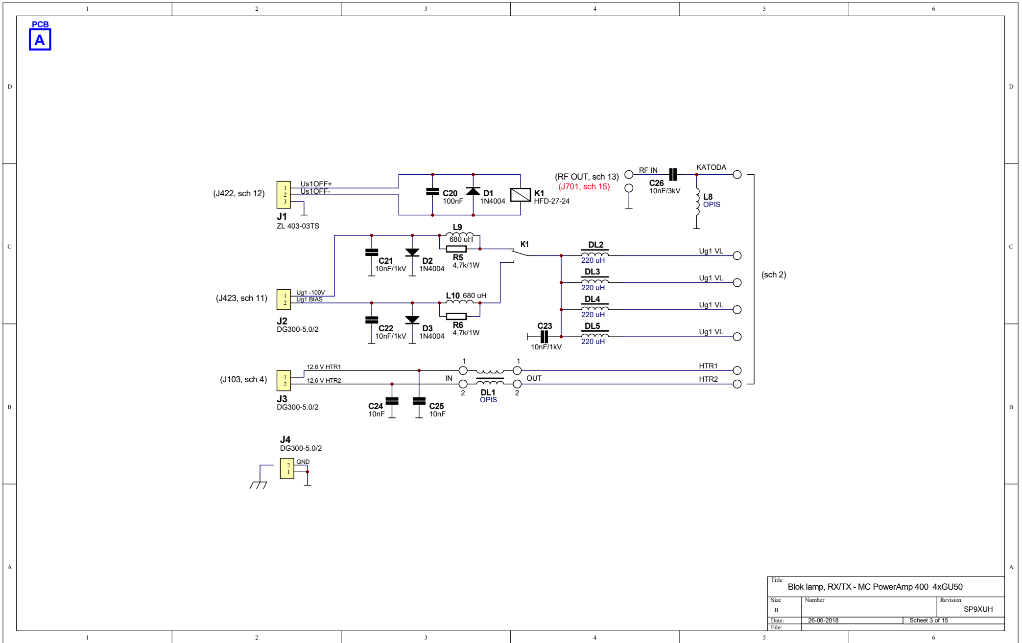
Schemat 3 - Blok lamp.
