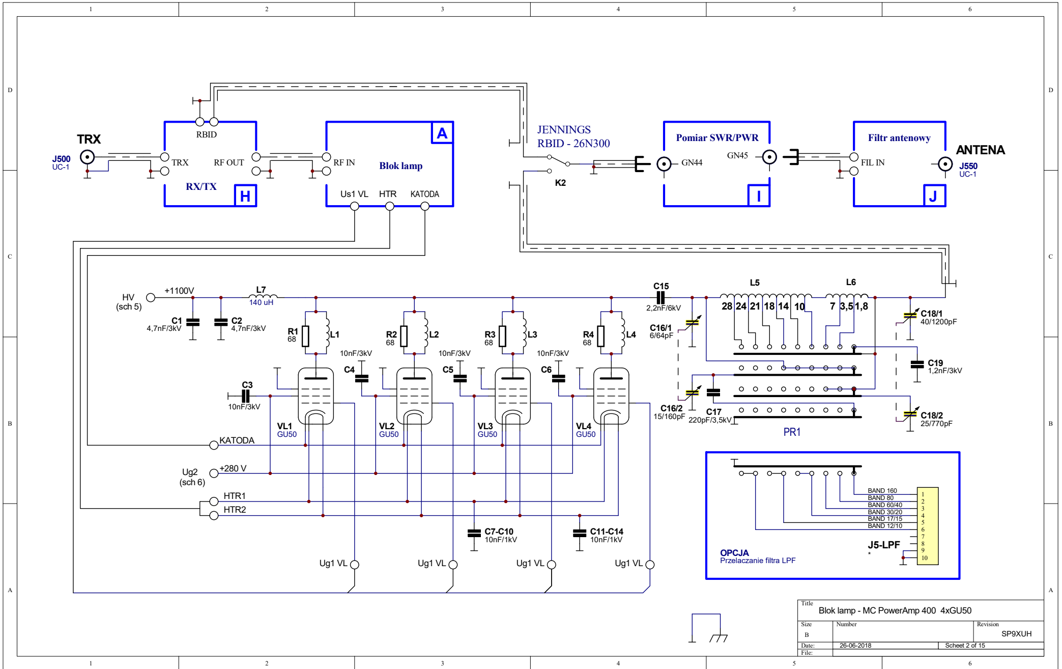
Schemat 2 - Blok lamp.
