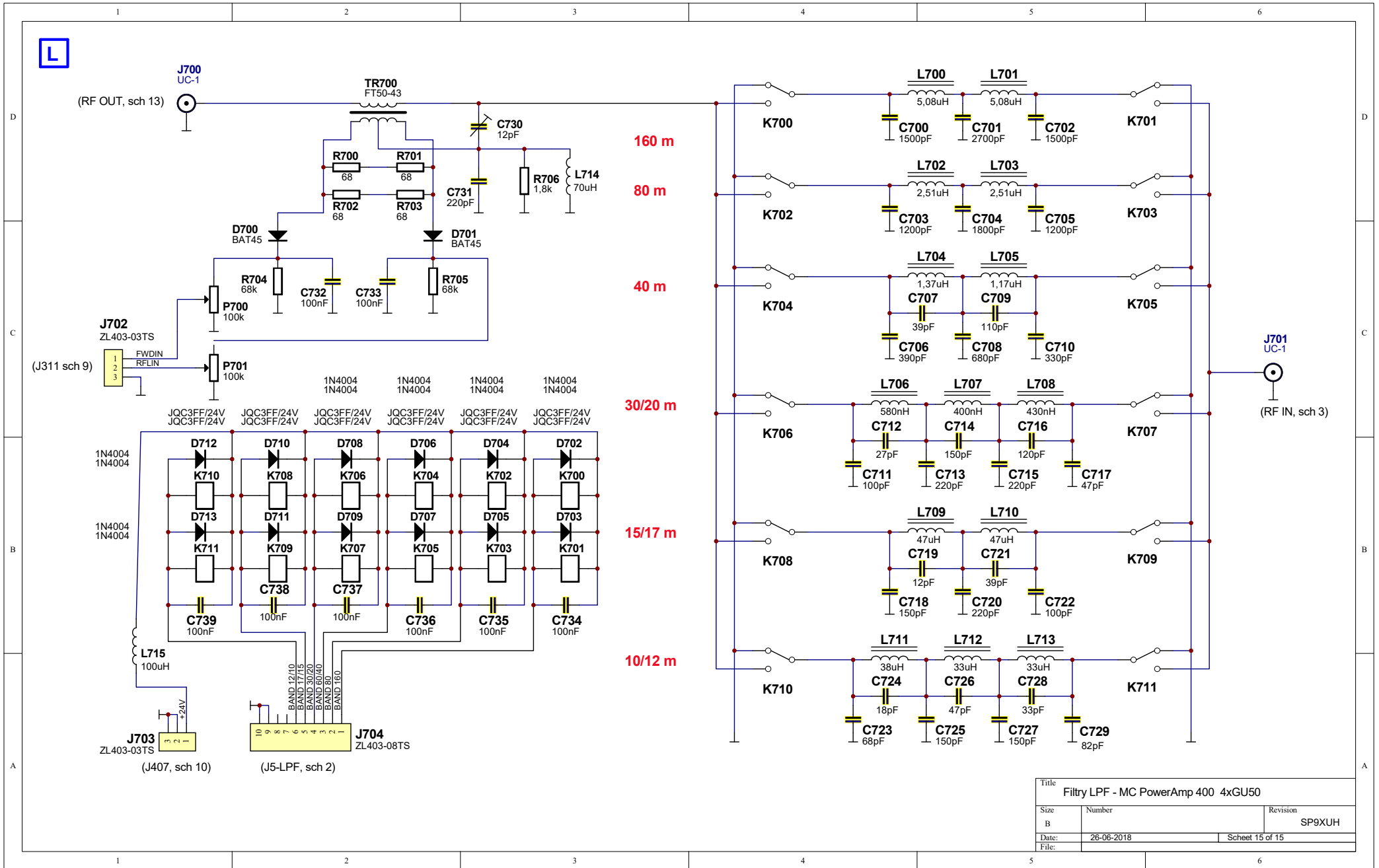
Schemat 15 - Filtry LPF.
