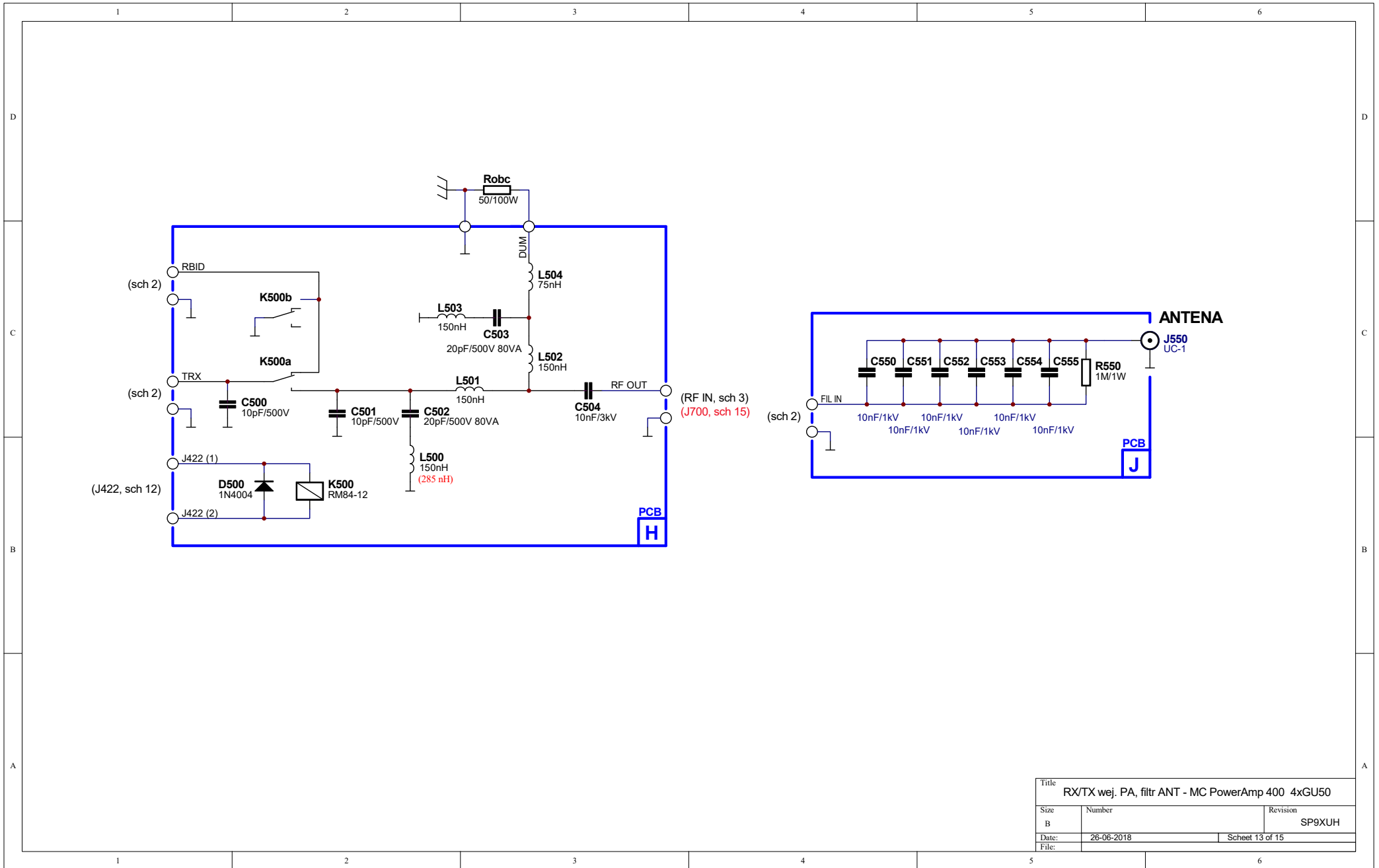
Schemat 13 - Przełączanie RX/TX; wejście PA.
