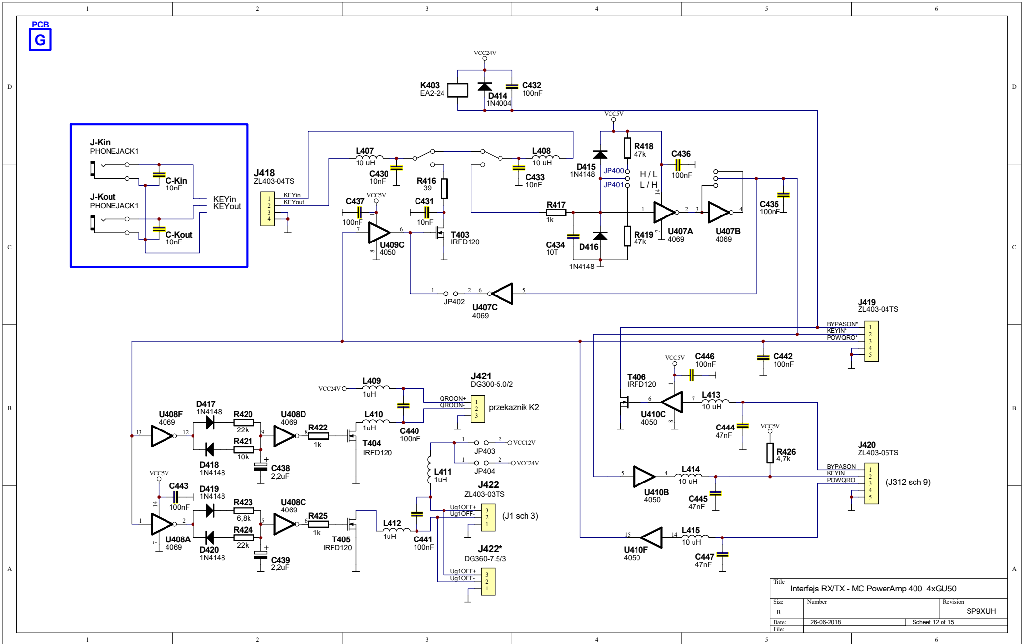
Schemat 12 - Przełączanie RX/TX; wyjście PA.
