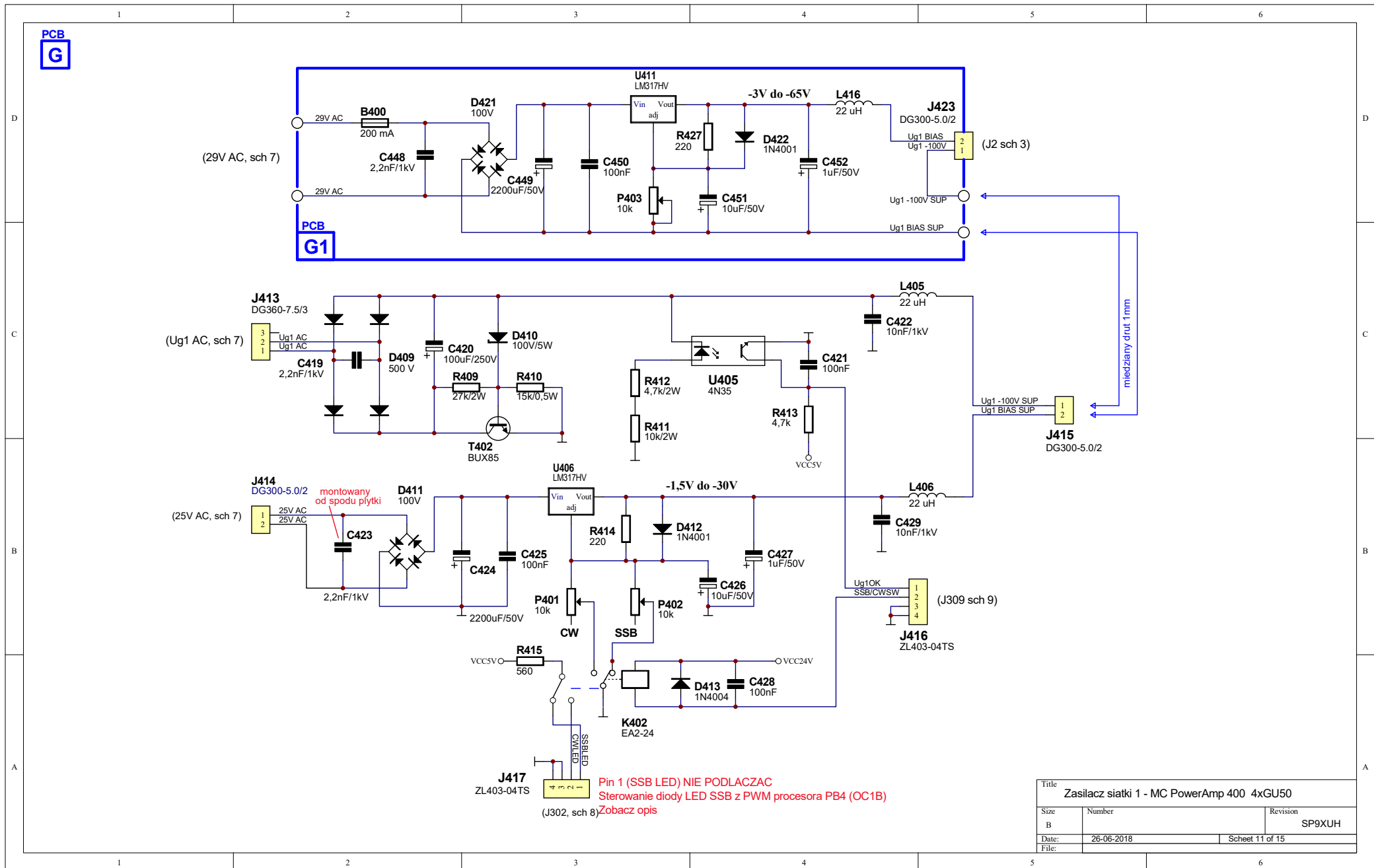
Schemat 11 - Zasilacz siatki sterującej.
