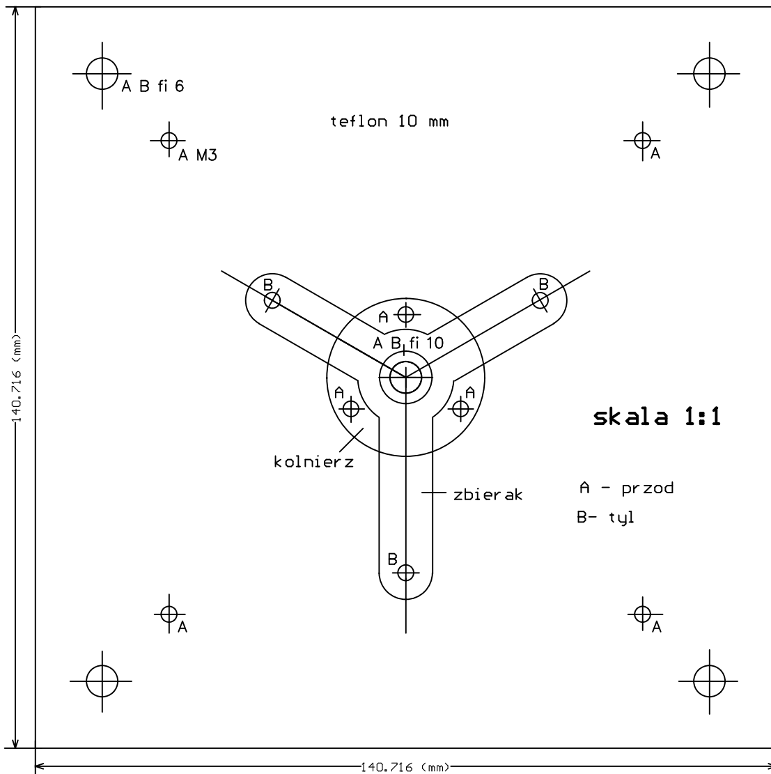
Rys. B-5-5 Elementy kondensatora antenowego filtra PI – I arkusz.
